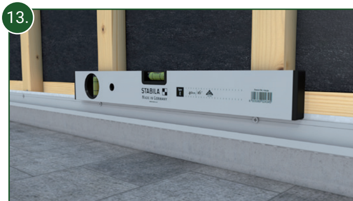
13. Achten Sie bei der Montage des Aluminium-Startprofils bitte auf eine exakte, horizontale Ausrichtung!
