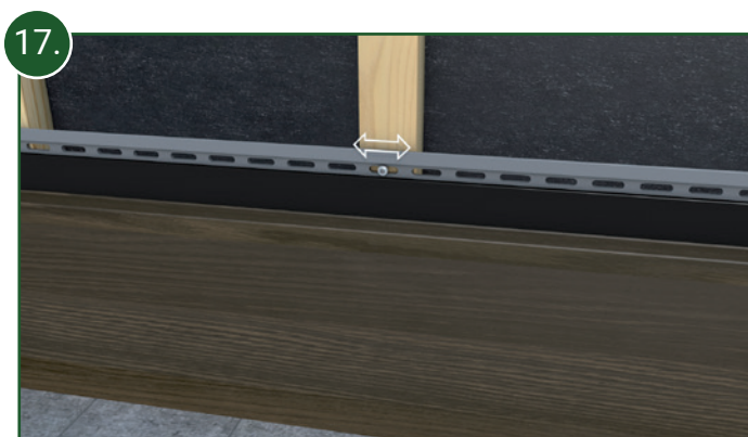
17. Die Verschraubung der Fassadenprofile mit der Traglattung erfolgt mittig durch die in den Federbereichen eingebrachten Langlöcher mittels der Fassadenschrauben.
