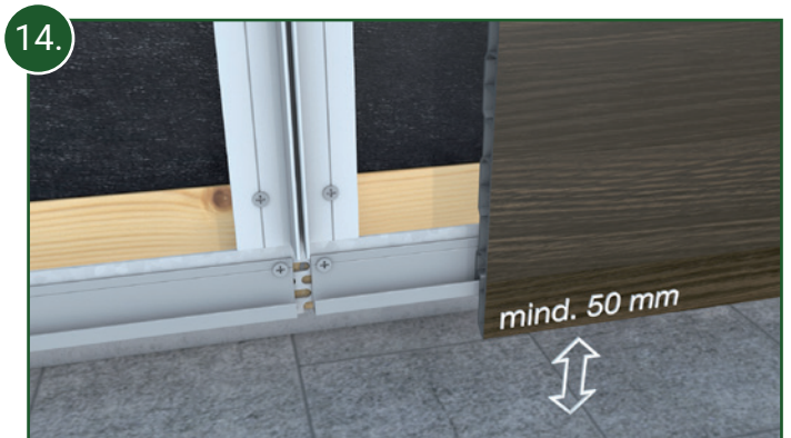
14. Die Montage der Fassadenprofile beginnt am unteren Fassadenrand, indem das erste Fassadenprofil gemäß Skizze in das Aluminium-Startprofil eingehängt wird. Bitte beachten Sie den Mindestabstand Unterkante Fassadenprofil von 50 mm zum Bodenniveau.
