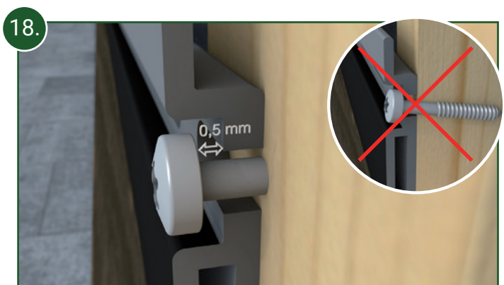
18. ACHTUNG: Die Fassadenschrauben dürfen nur so fest eingedreht werden, dass sich das Fassadenprofil nach der Verschraubung noch schieben lässt! Zudem dürfen die Schrauben nicht schräg eingebracht werden.
