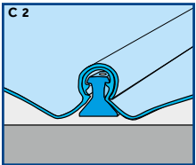
Befestigung der FASTLOCK®-Platten mit Topclips auf dem Balken
