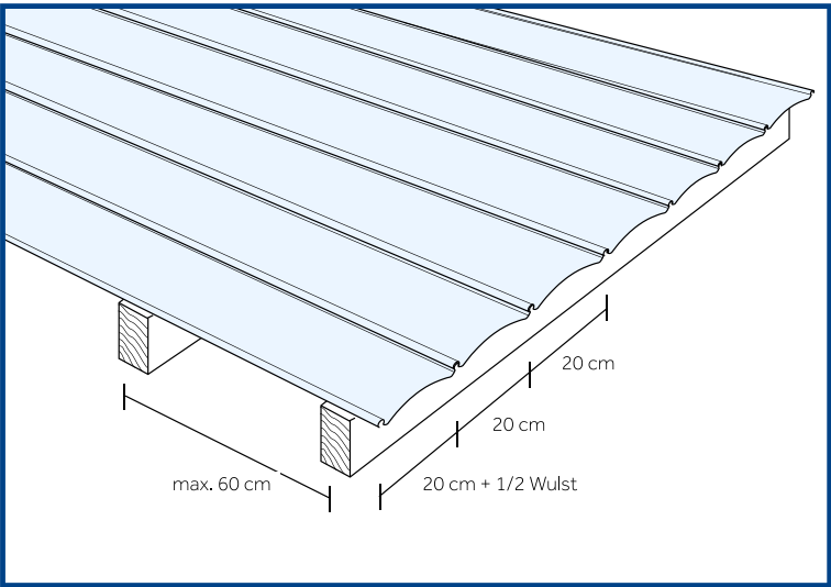
Befestigung der FASTLOCK®-Platten mit Topclips auf dem Balken
