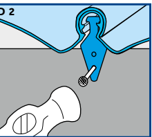
Befestigung der FASTLOCK®-Platten mit Lattenbeschlag seitlich am Balken
